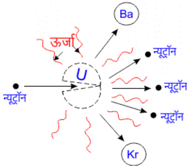
नाभिकीय विखंडन
